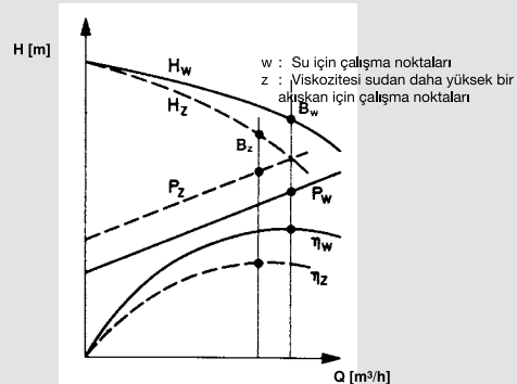
Çalışma noktalarının viskoziteye bağlı olarak değişimi
